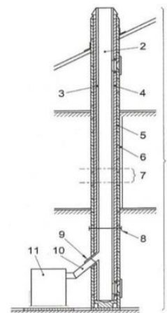
Bestandteile und Nebenelemente eines Kamins
